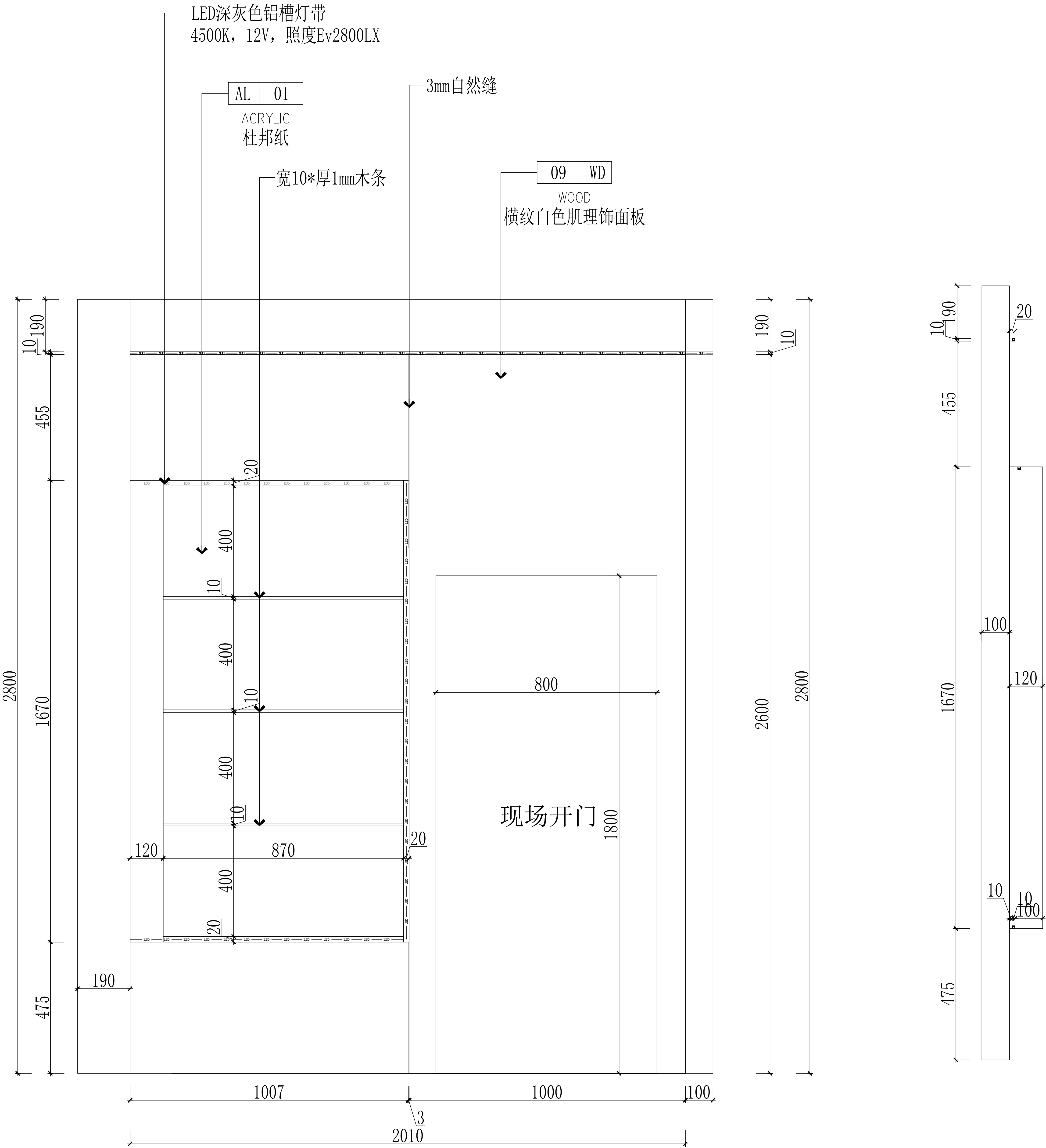
D 立面图
