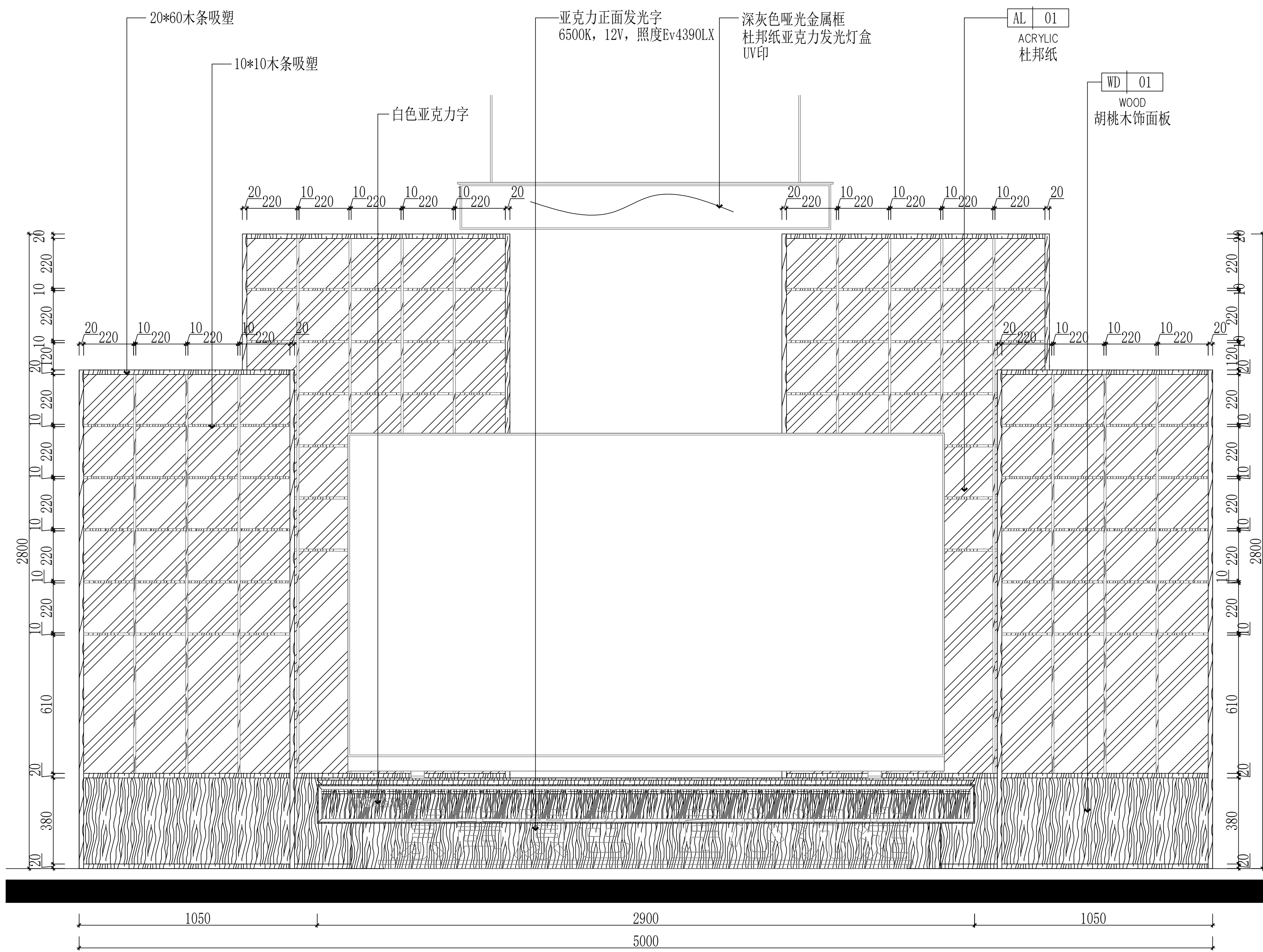
立面图
