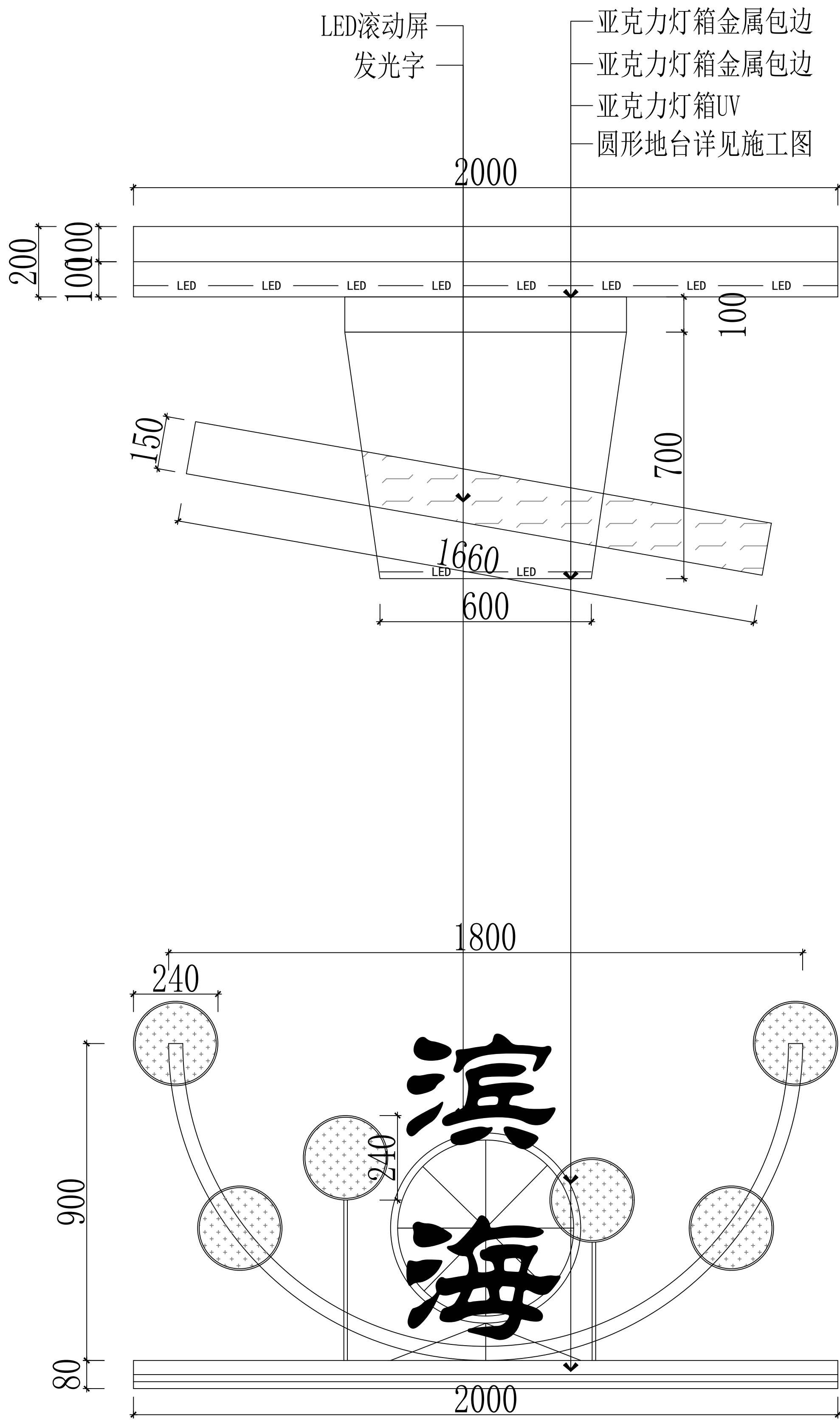
E 立面图
