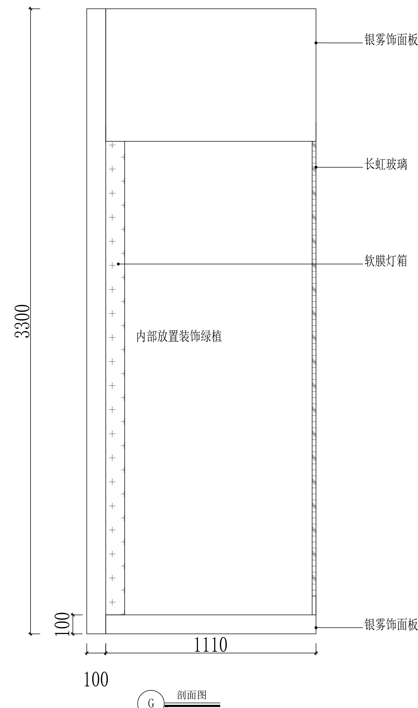
G 剖面图
