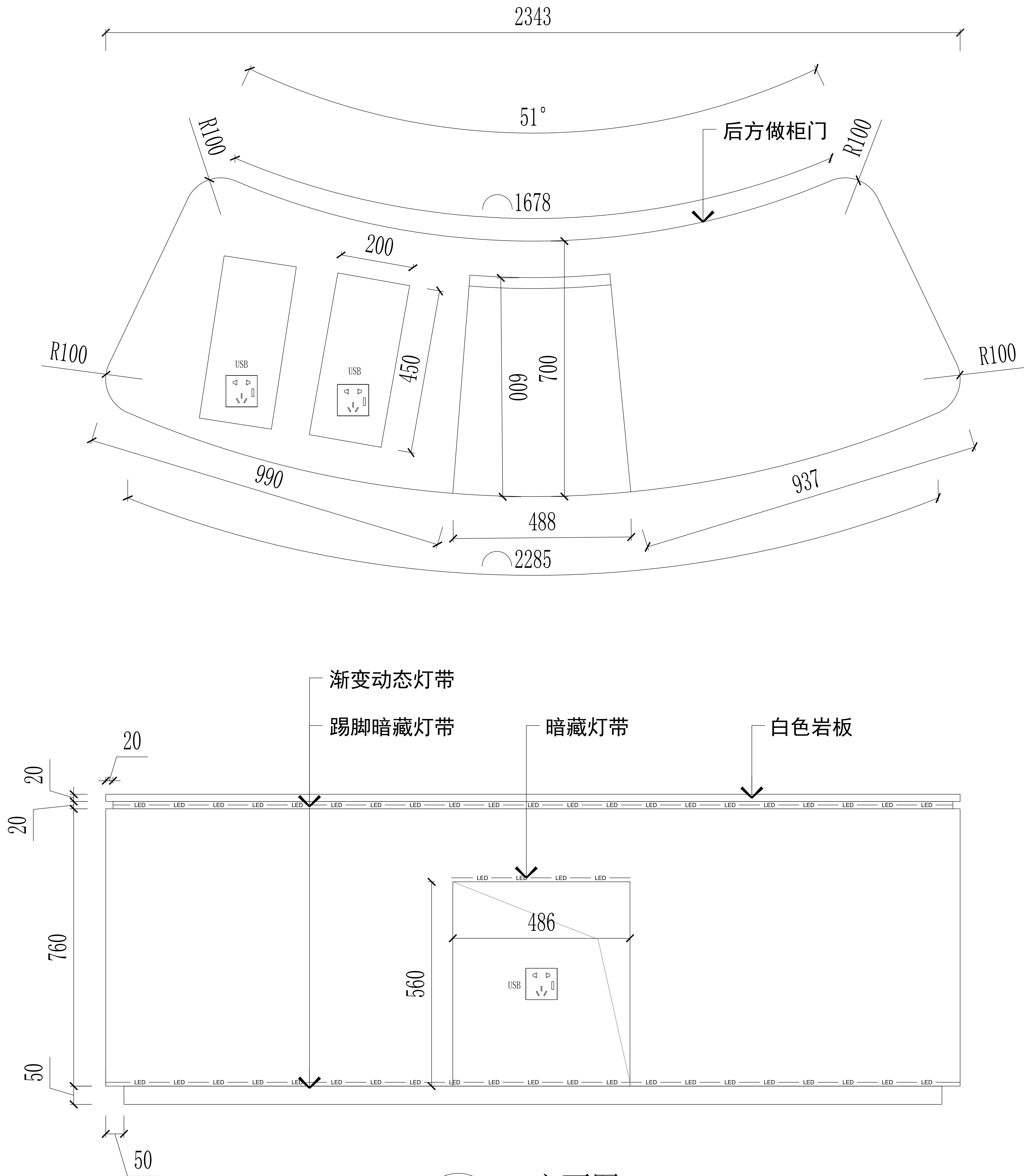
03 立面图
