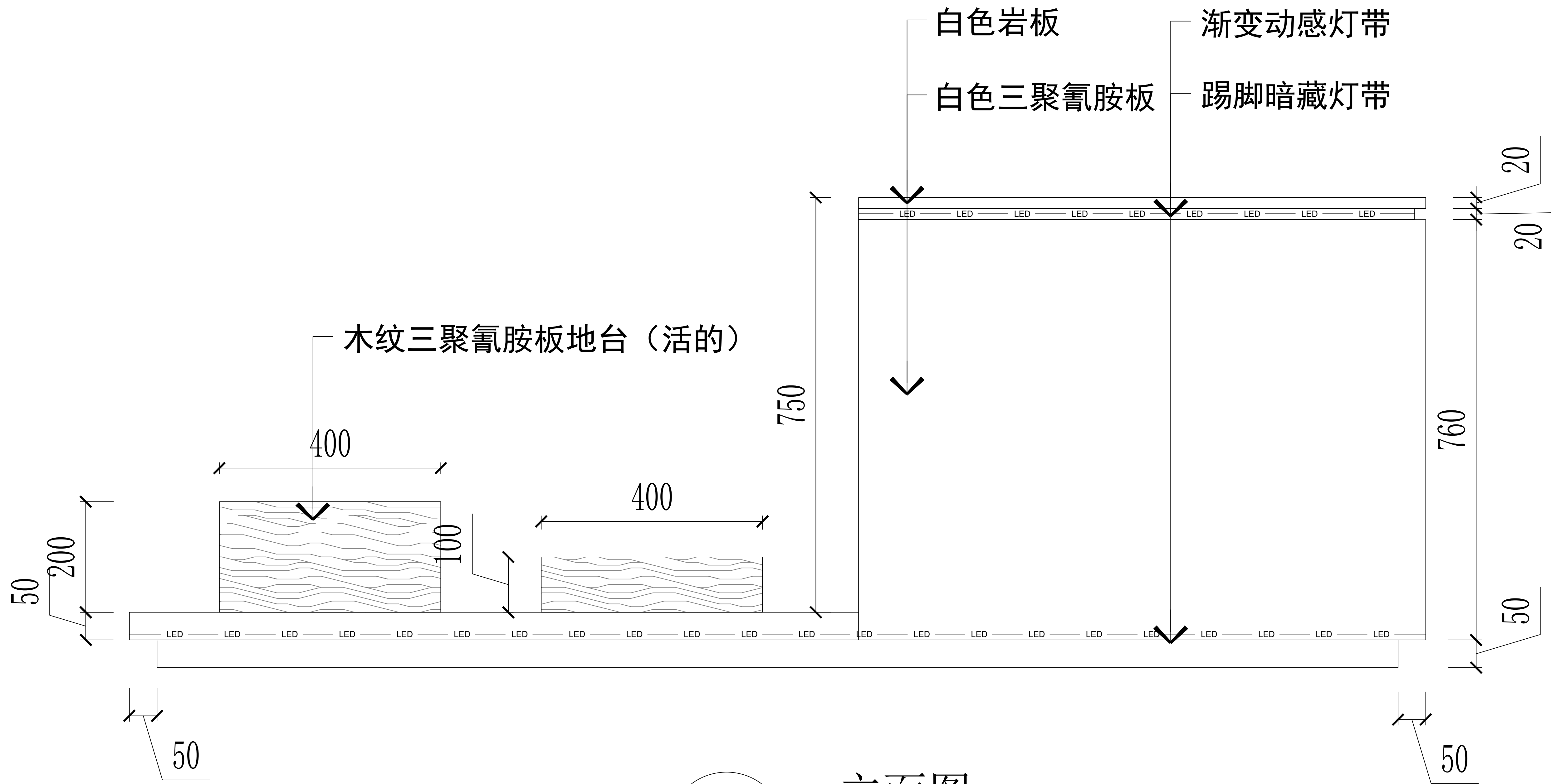
02 立面图
