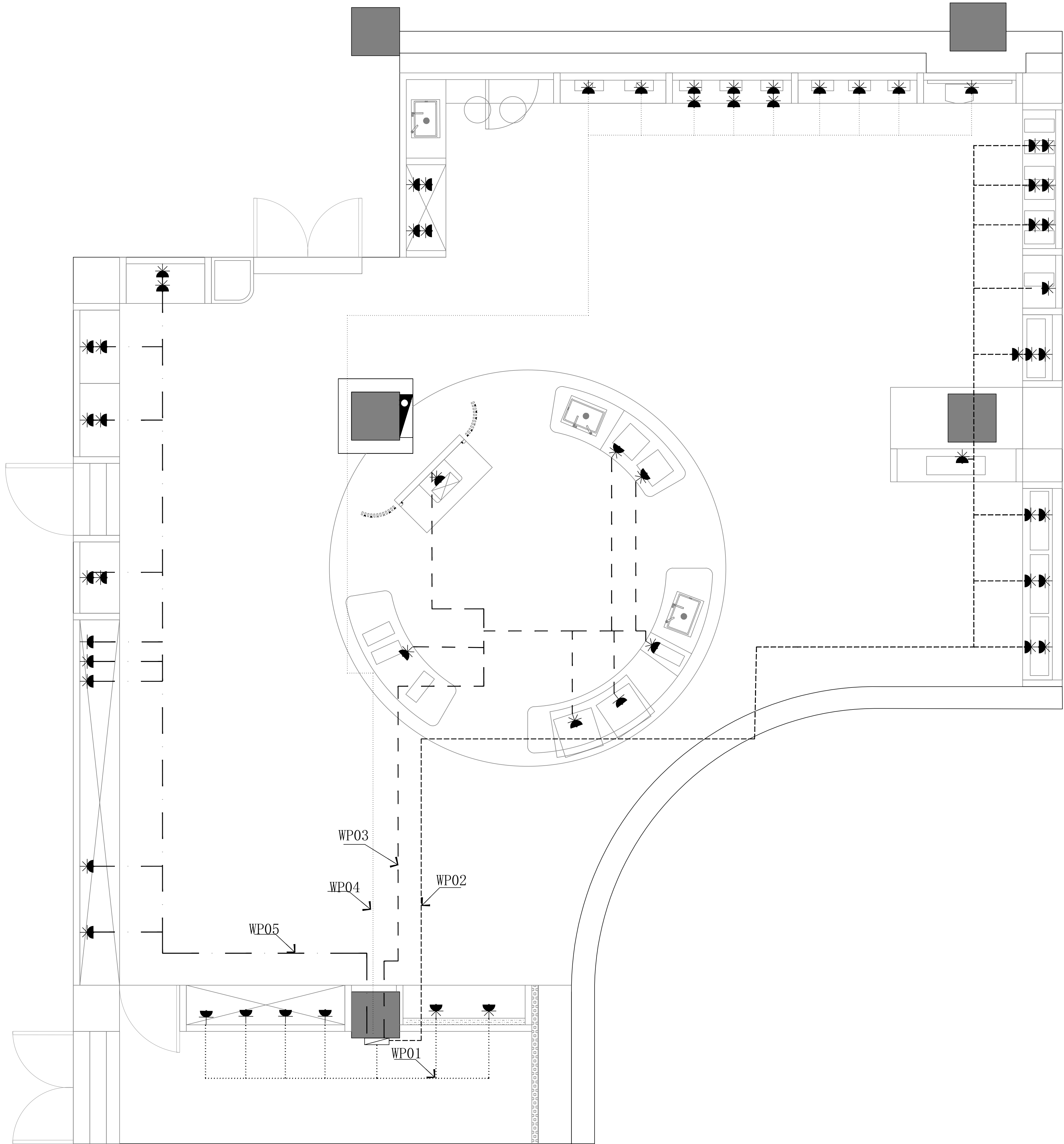
插座连线图
