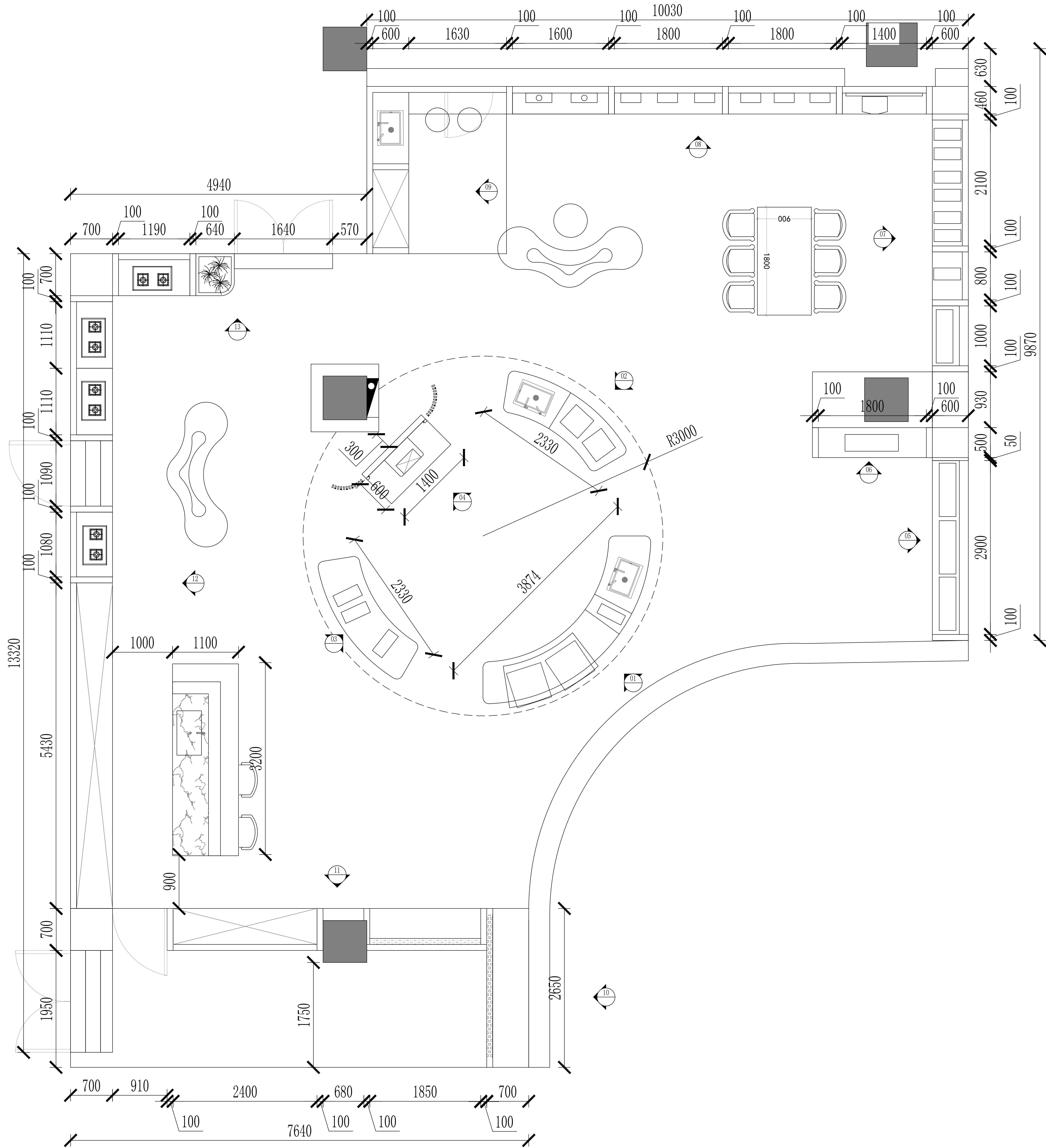
平面索引图
