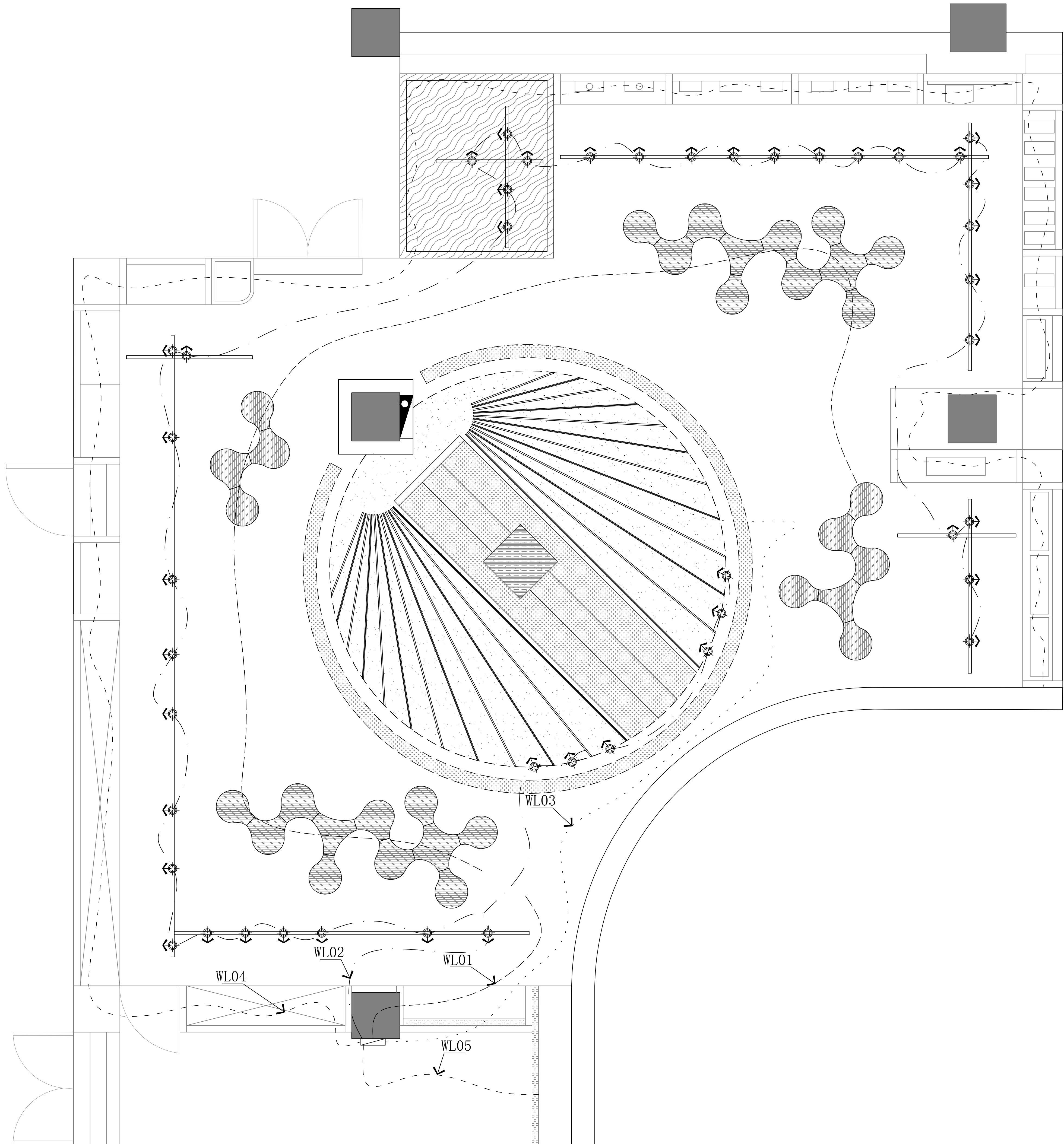
灯具连线图
