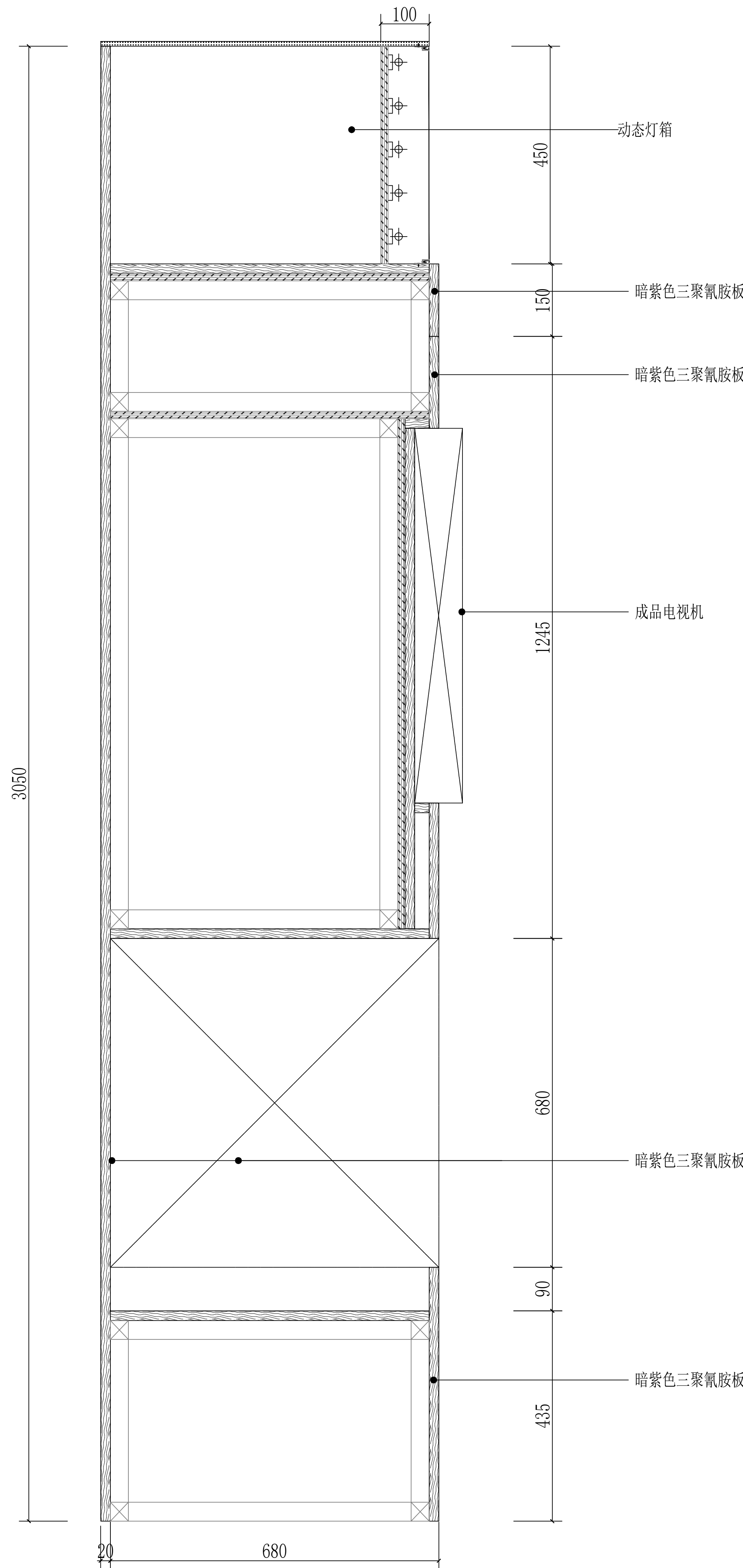
R 剖面图
