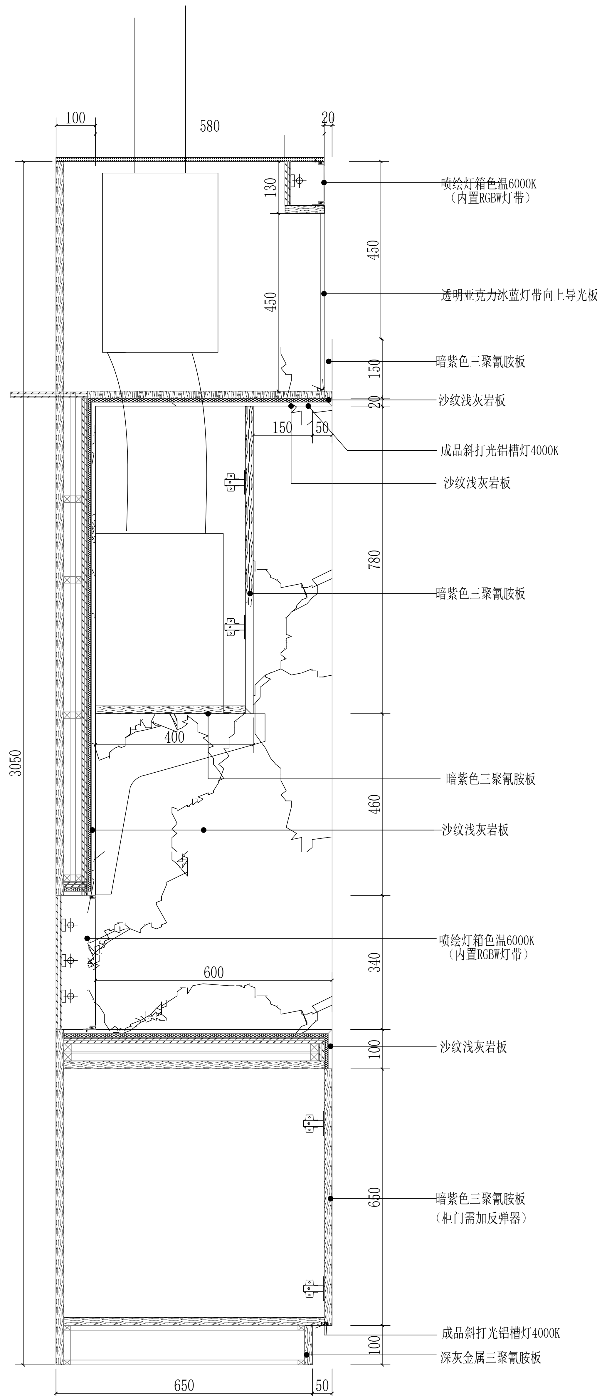
Q 剖面图
