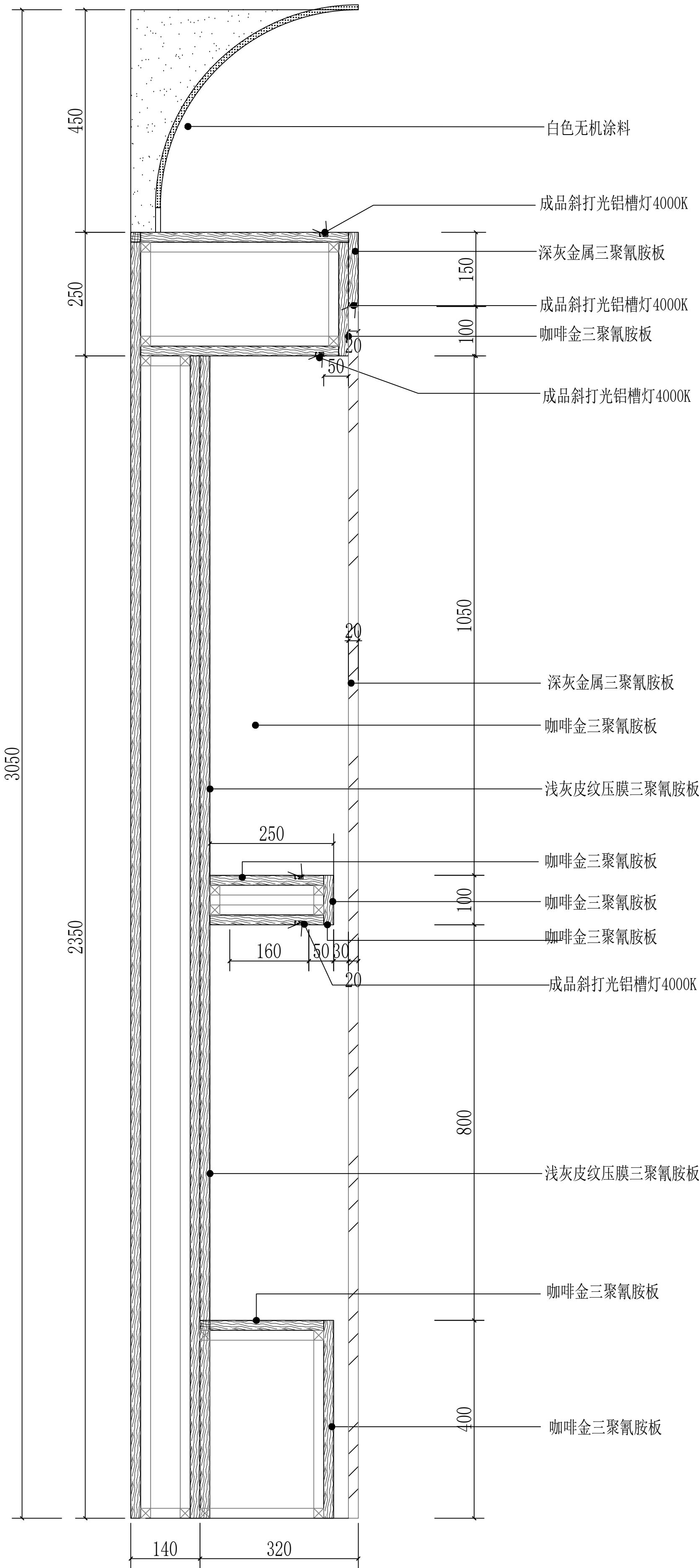
J 剖面图
