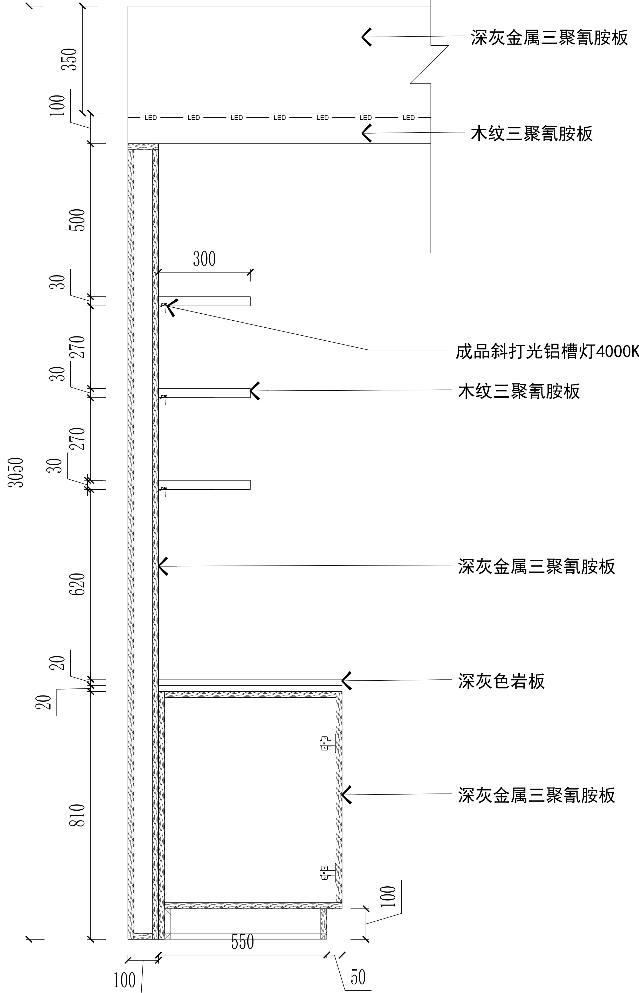
L 剖面图
