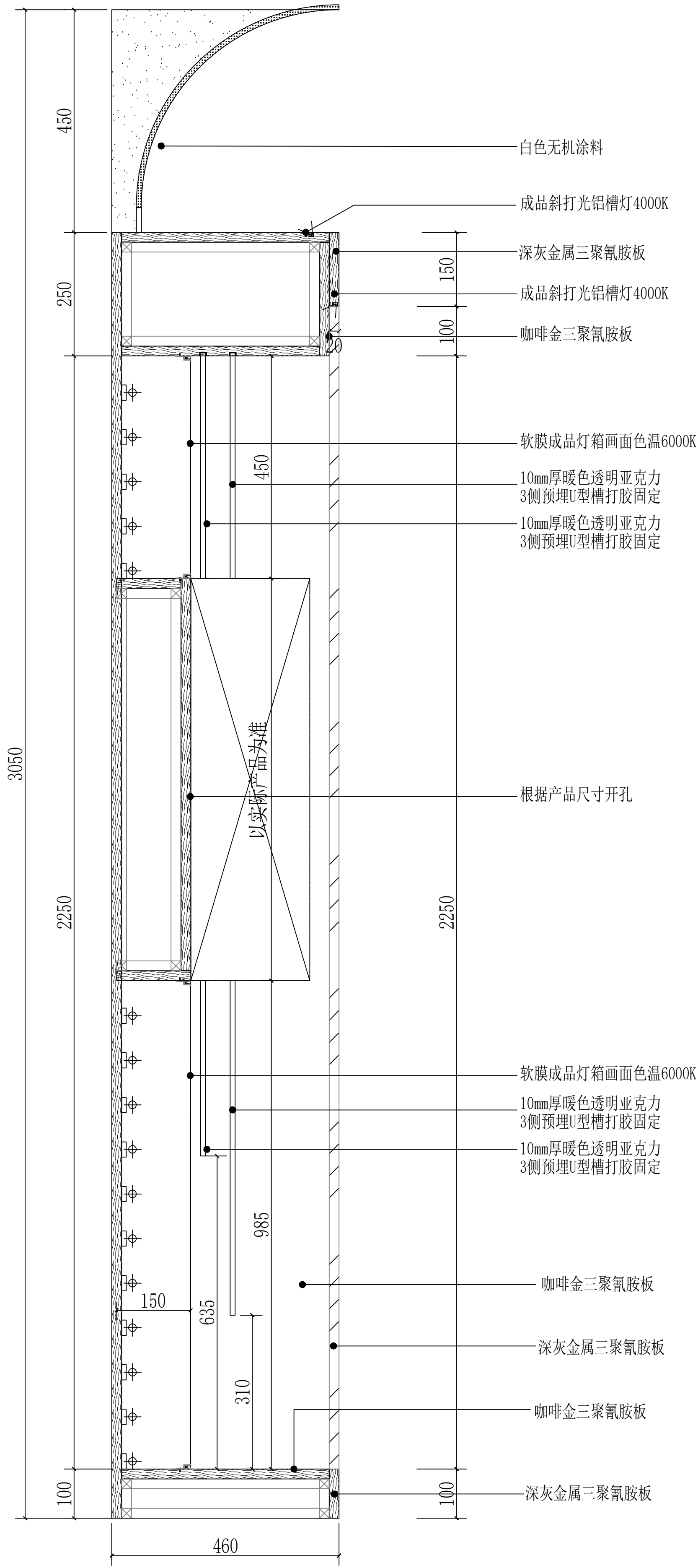
K 剖面图
