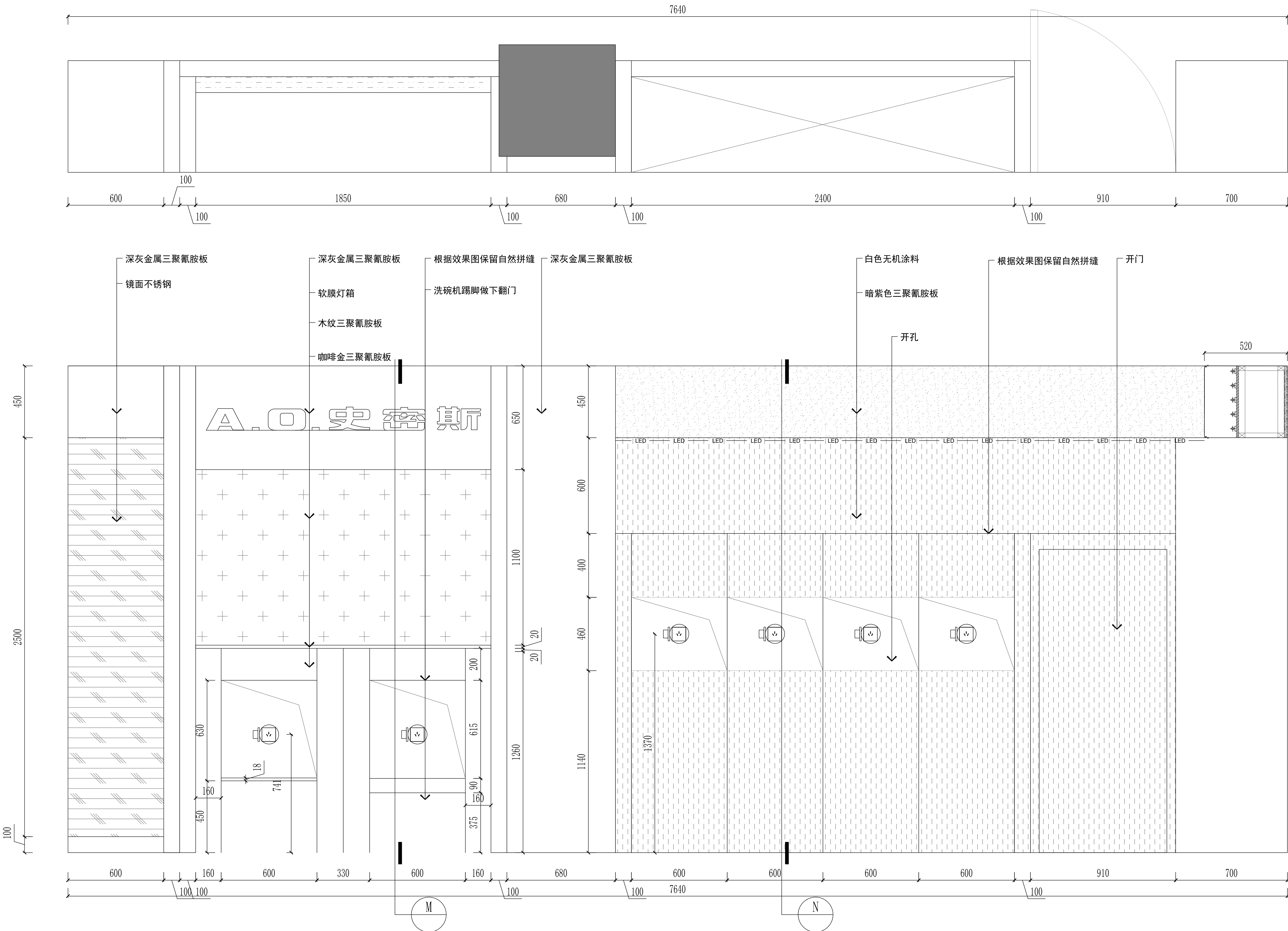
11 立面图
