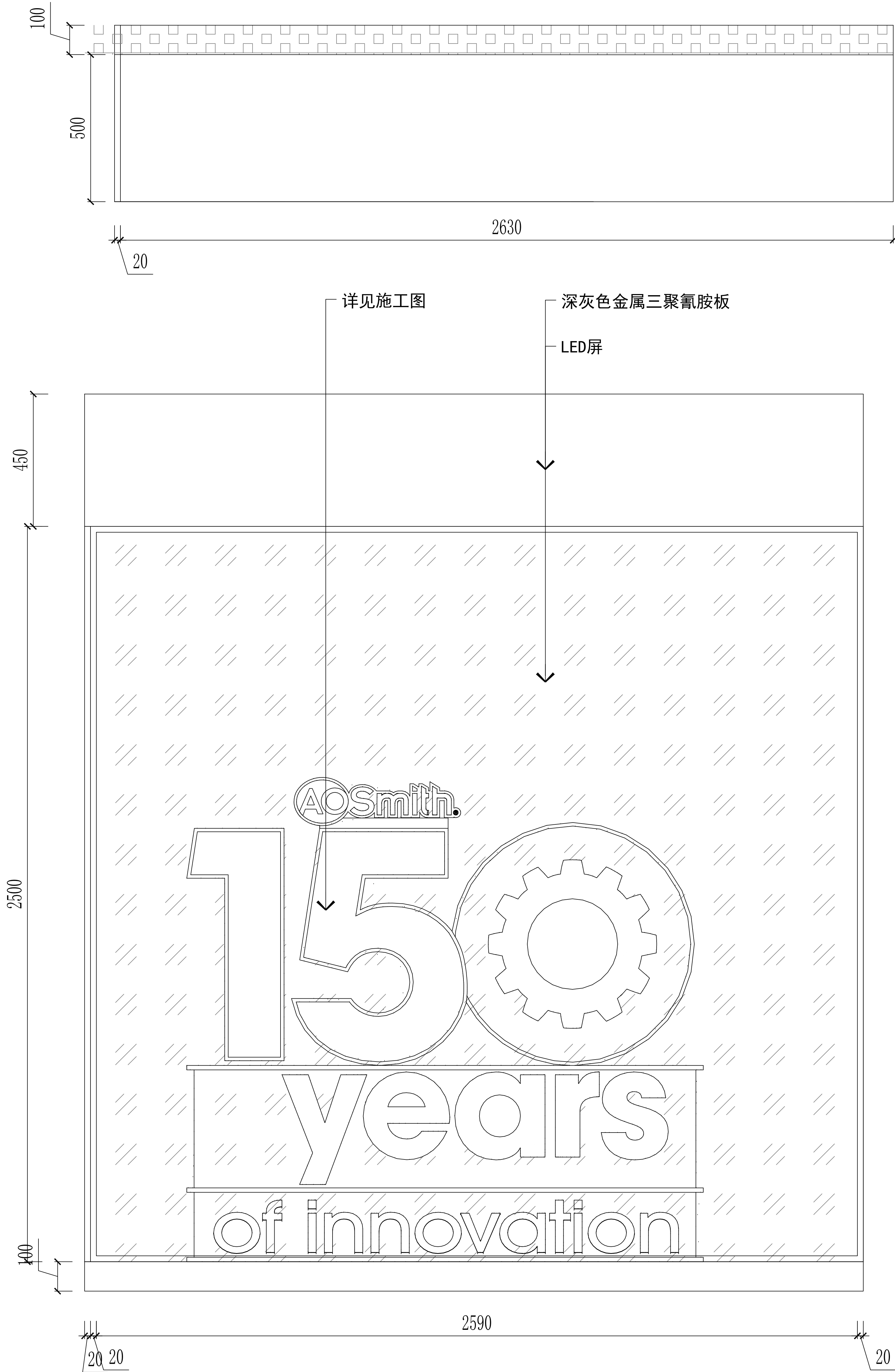
10 立面图
