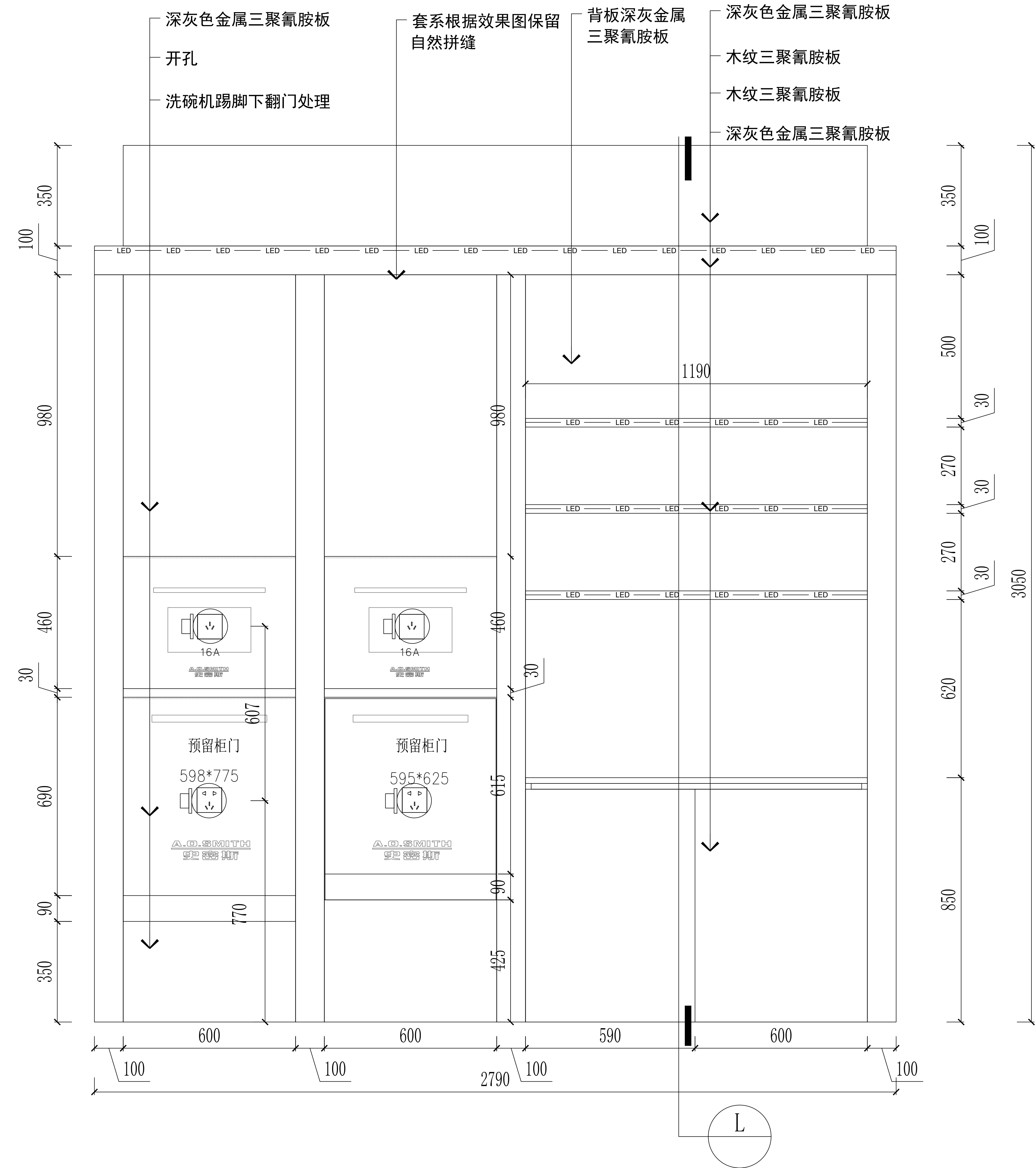
09 立面图
