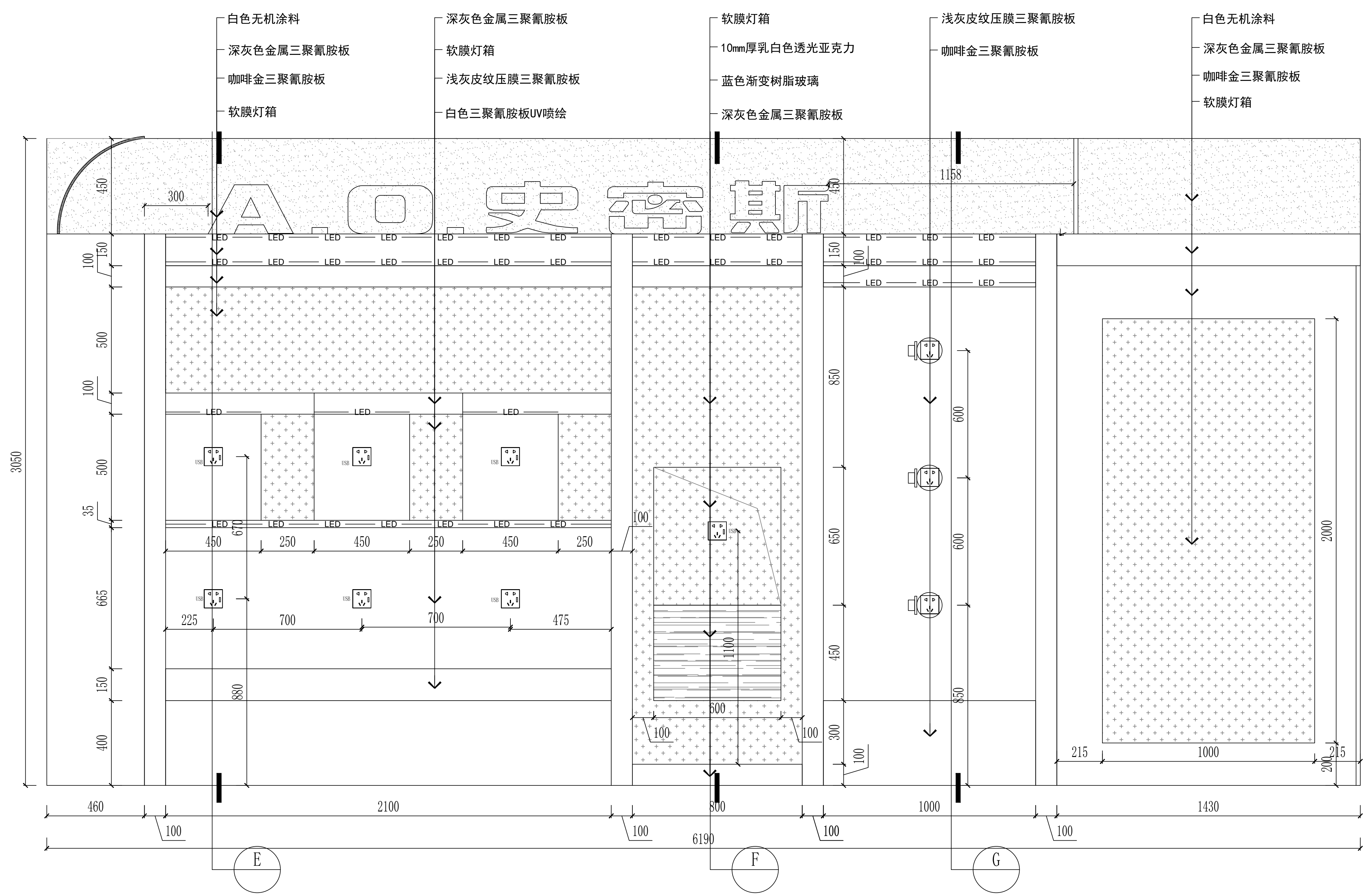
07 立面图
